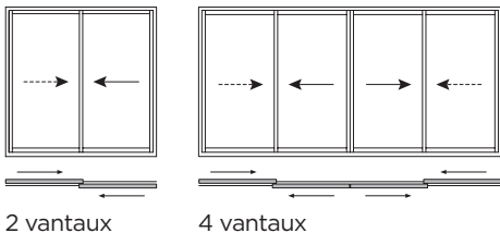
2 vantaux 4 vantaux
