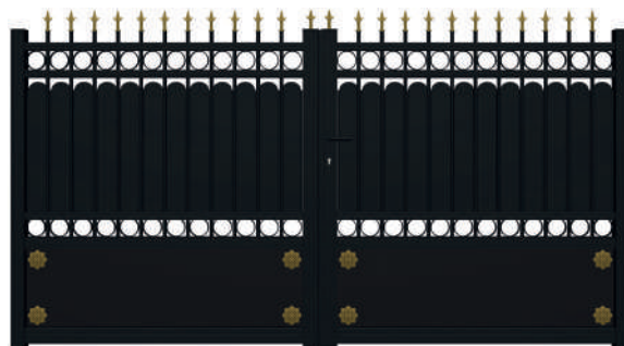
2 vantaux : barreaux Ø 20 mm, tôle ép. 3 mm, feston ép. 2 mm, fers de lance fleur de lys et marguerites Coloris : noir foncé RAL 9005, bi-coloration sur les ornements
