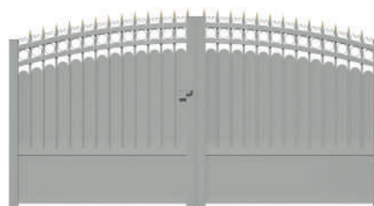
2 vantaux Albinoni : forme bombée E, barreaux Ø 20 mm, tôle ép. 3 mm, feston ép. 2 mm, fers de lance pointe et rangée de petites volutes sur traverse haute Coloris : gris clair RAL 7035, bi-coloration sur les ornements
