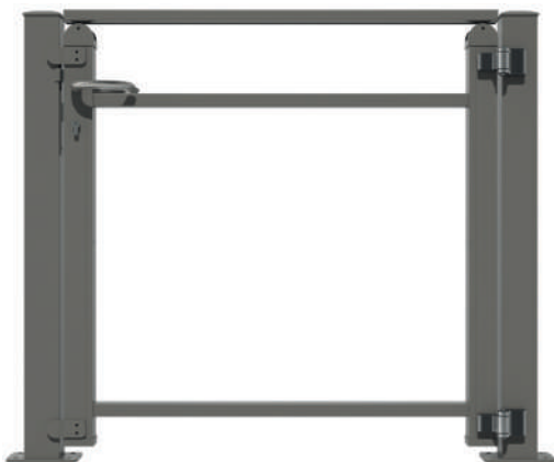
Portillon Béring : sans lisse et verre transparent Coloris : gris quartz RAL 7039
