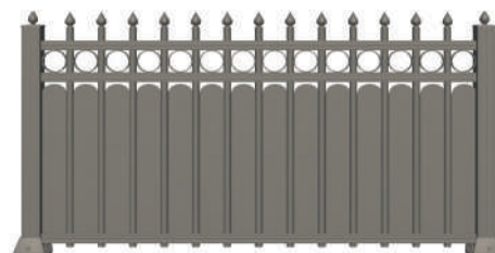
Clôture Albinoni : barreaux Ø 20 mm et tôle feston ép. 2 mm
