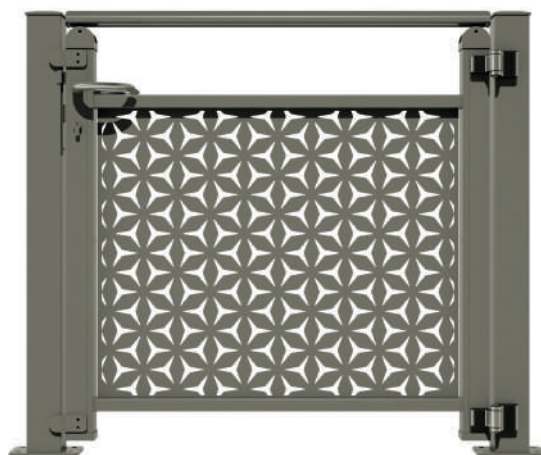
Portillon Bosphore : sans lisse et tôle personnalisée motif Eolienne Coloris : gris quartz RAL 7039
