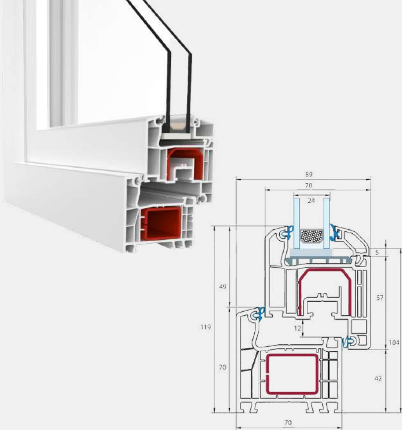
Fenêtre PVC coulissant série PVC WINSLIDE
